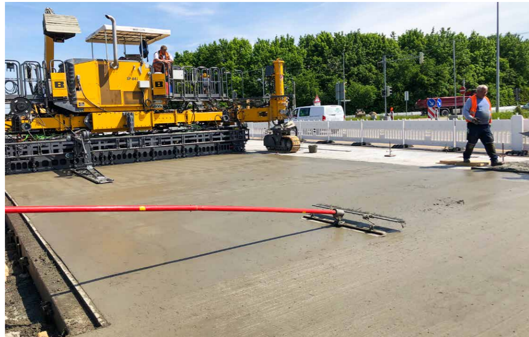
Aufbringen des Besenstrichs
