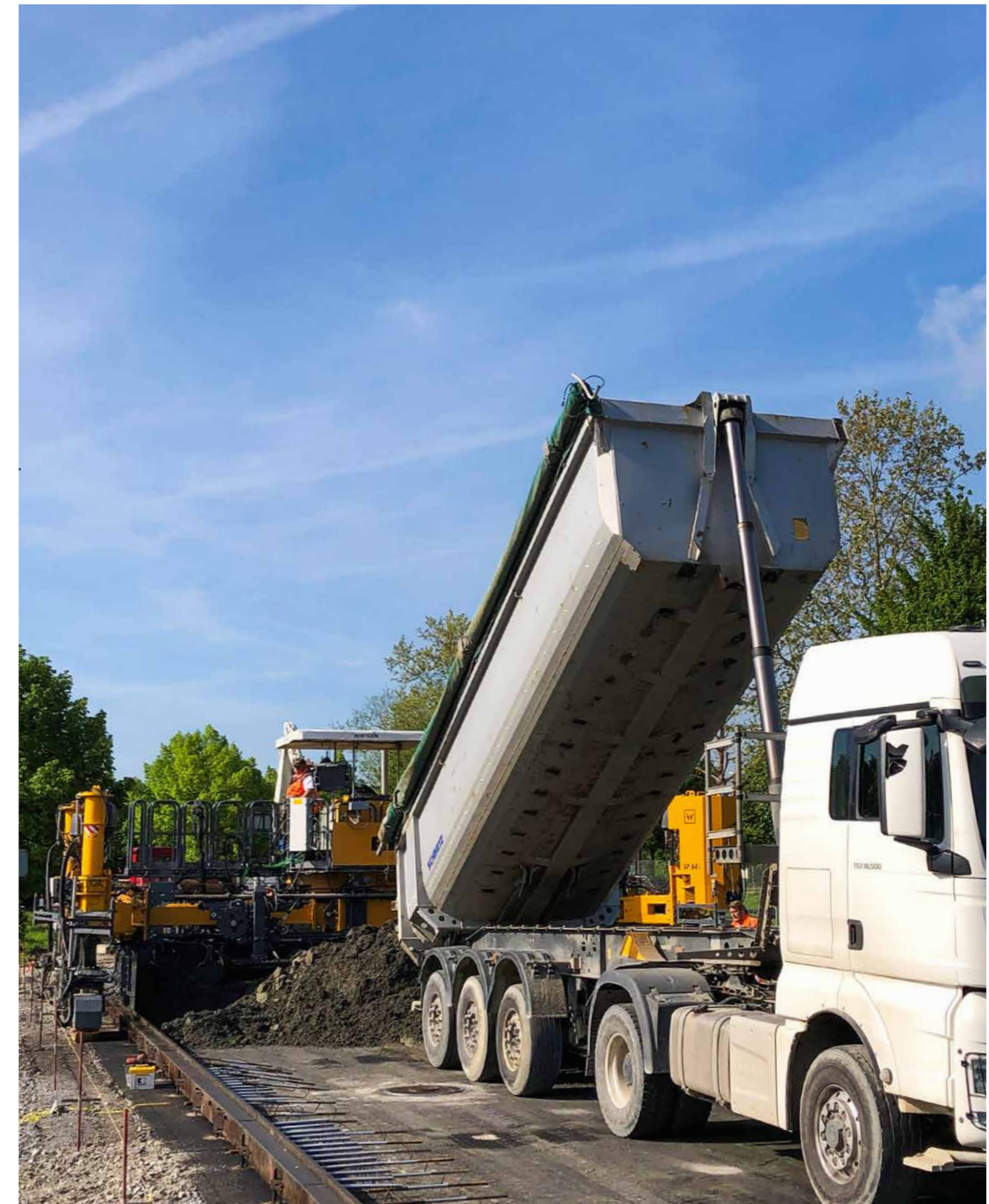
Betoneinbau mit Beton-Straßenfertiger in der Konsistenzklasse C1
