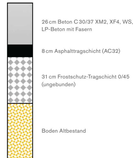
Aufbau Gesamtquerschnitt Daimler-Knoten
